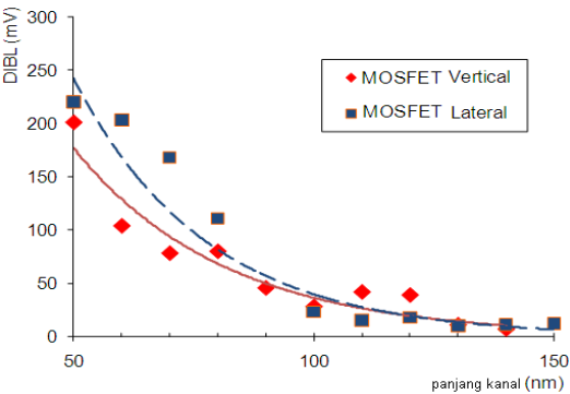
Gambar 1. Tren DIBL untuk MOSFET
